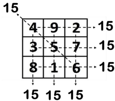
Fig. 4 Equilibrio matematico
